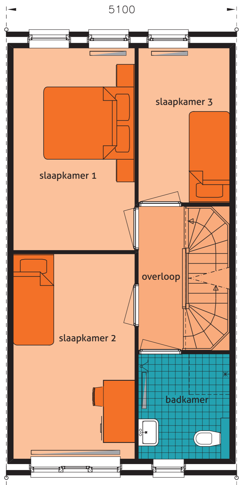
getekend is 1e verdieping (a)
