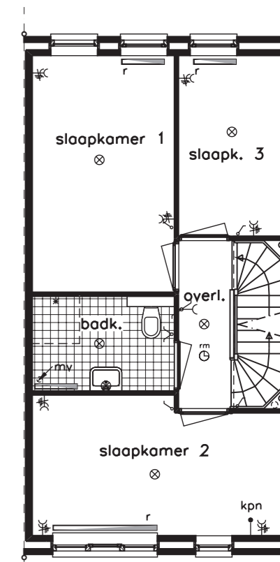
1e verdieping (c)
