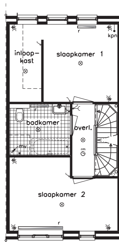
1e verdieping (d)
