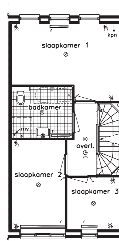
1e verdieping (b)
