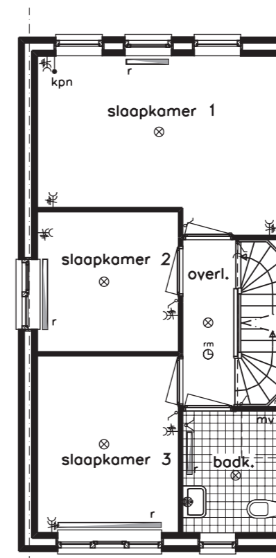
1e verdieping (e)
